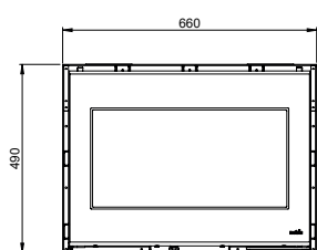
Technische tekening Efrem 700.49
